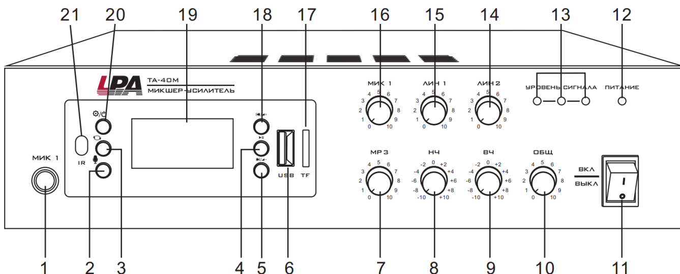
Рис. 3.2. Схема расположения средств управления LPA-TA-40M
