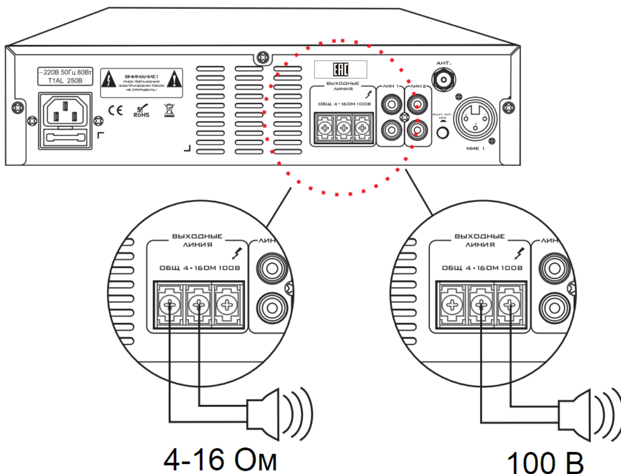
Рис. 2.2. Схема подключения громкоговорителей к LPA-TA-40M
