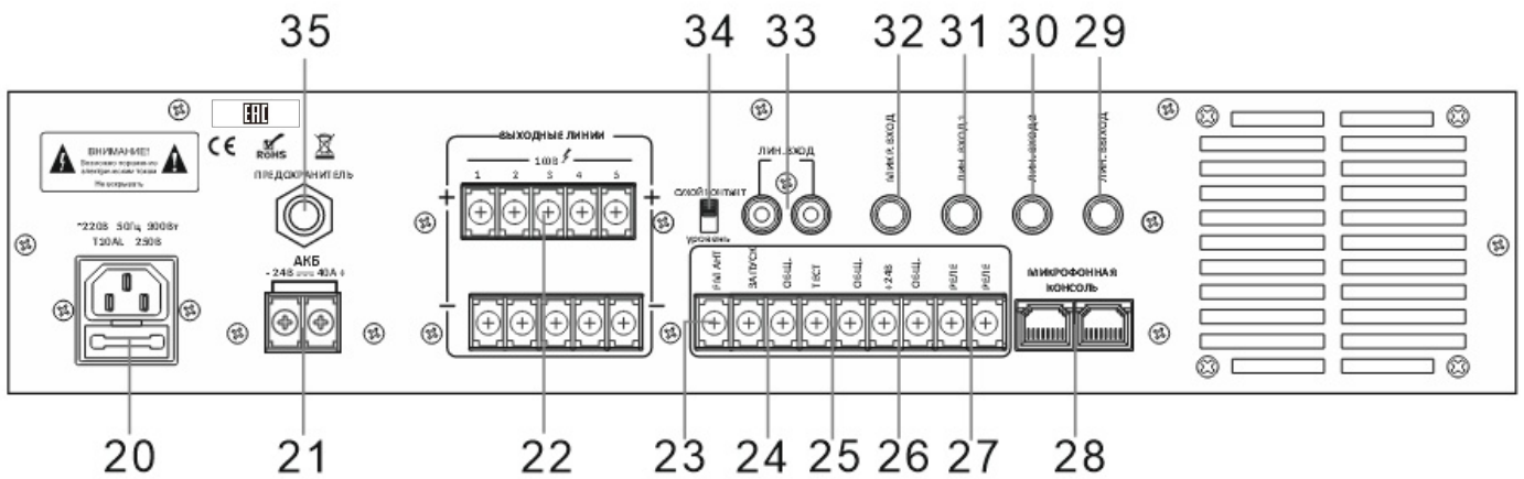
Рис. 1.3. Задняя панель
