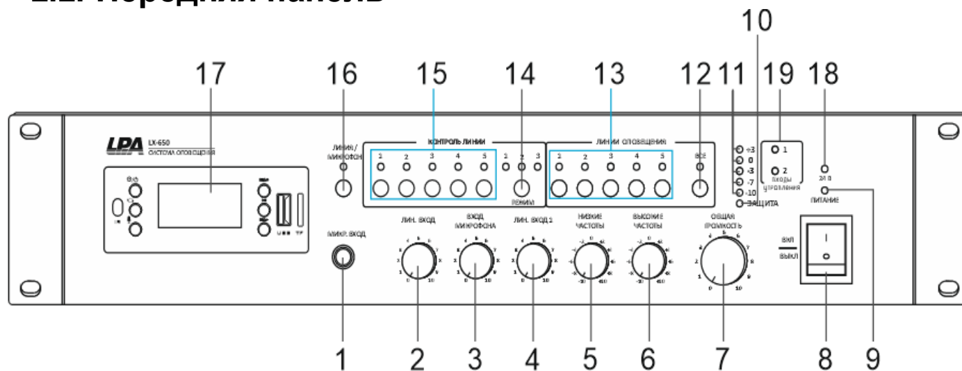
Передняя панель
